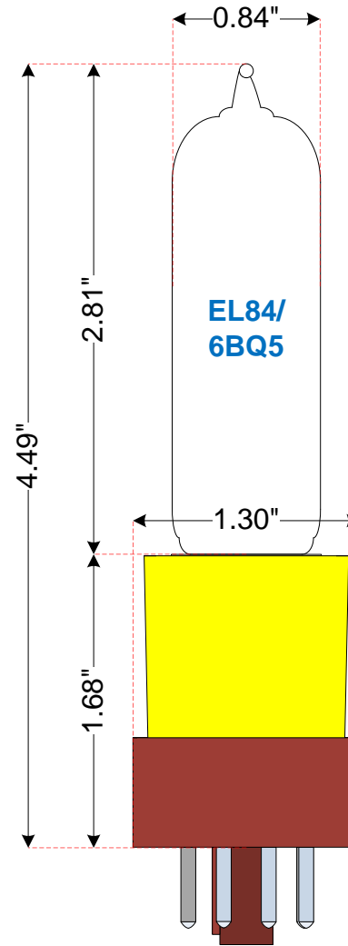
Dimensions for: YJSHORT YJUNI
