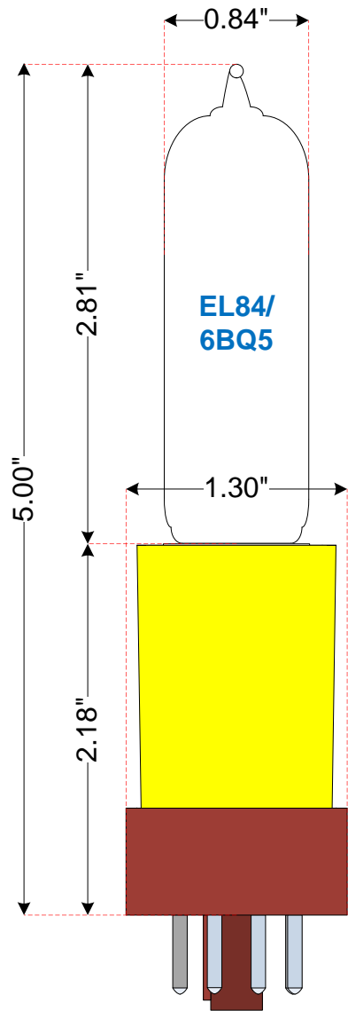
Dimensions for: YJS YJC YJ20 YJ7591
