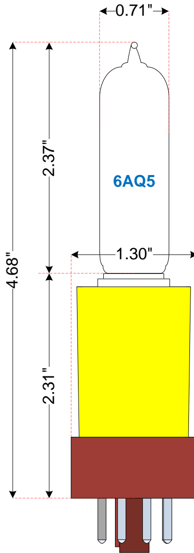
Dimensions for: YJNOS
